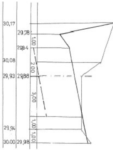
1+006
